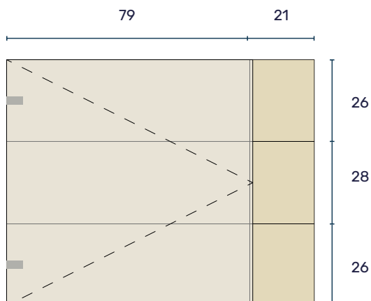
BM108 L.100 cm H.80 cm P.9 cm
