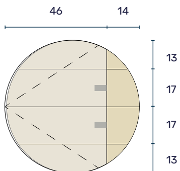
BM60D Ø 60 cm P.9 cm
